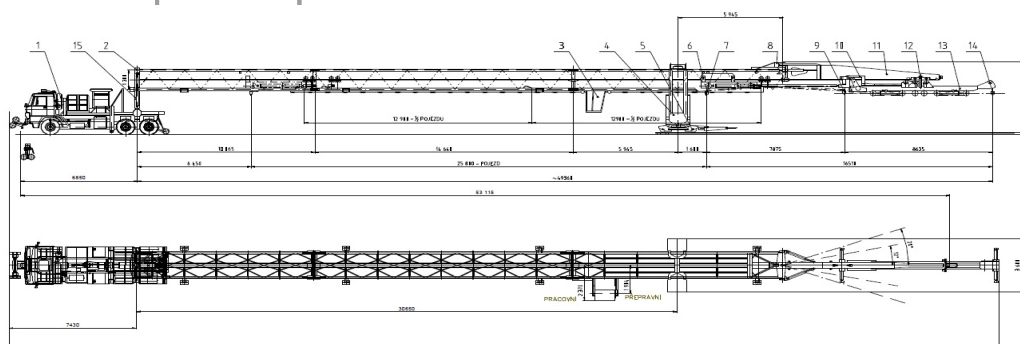
1-tahač s nástavbou T815 Z; 2-DÍL a; 3-kabina jeřábů; 4-sloup portálu; 5-podvozek portálu; 6-kočka č. 1; 7-závěs č. 1; 8-díl C; 9-závěs č. 2; 10-kočka č. 2; 11-díl D; 12-kočka č. 3; 13-kyvné rameno; 14-závěs č. 3; 15-štitník
